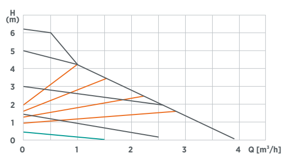
Kennlinie WITA Delta MIDI 60
