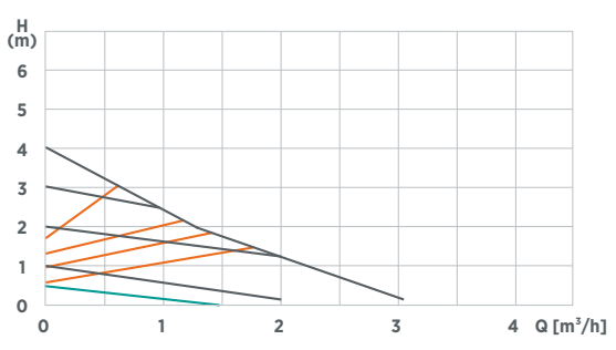
Kennlinie WITA Delta MIDI 40
